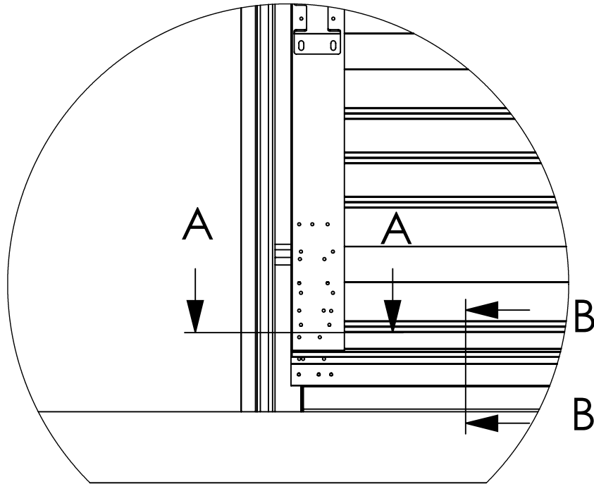
Detail rail en paneel bij vloer-waterkering
